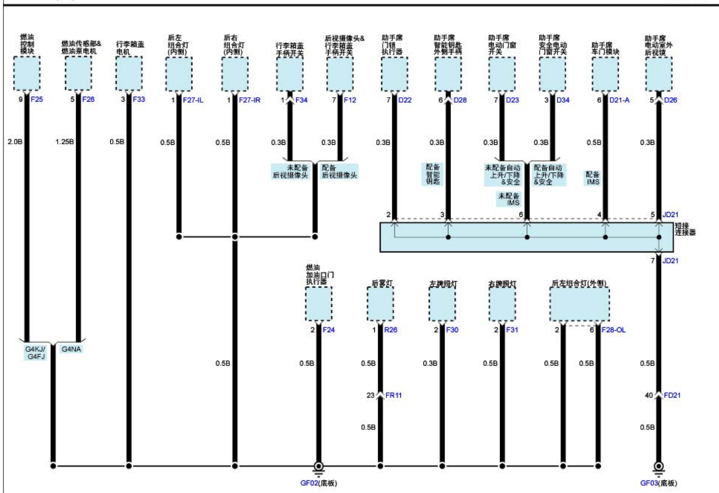
搭铁分布(14)
